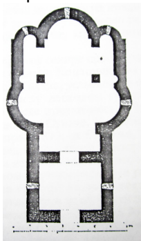
Црква Петруша - основа
